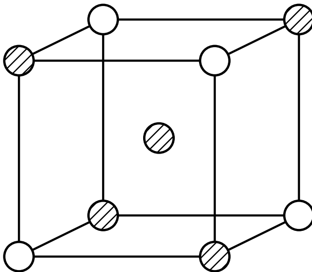
图 7 补全每个原子周围四面体的空缺位置（圆圈 O）以构成立方体，即给出强反射的 b.c.c. 格子
