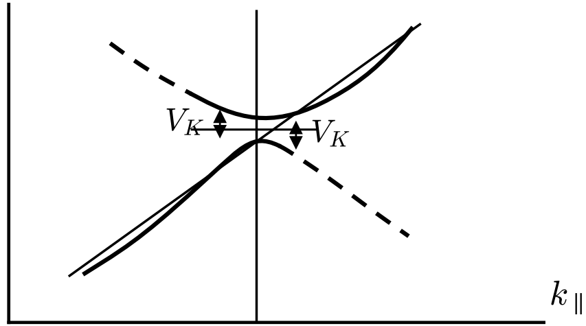
图 3 (原书图注仅 “ Figure 3 ” : 沿 k_{\parallel} 方向的恒能线, 自由电子交叉直线在区边界处劈裂, 能隙为 V_K )
