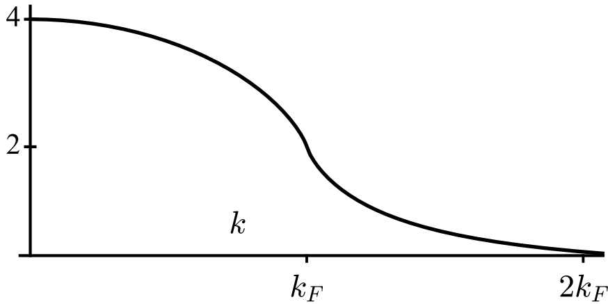
图 13 A_k 表达式中方括号内的函数随 k 的变化： k=0 处值为 4， k=k_F 处斜率无穷大，横轴标出 k 、 k_F 、 2k_F （原书图注仅作“Figure 13”）
