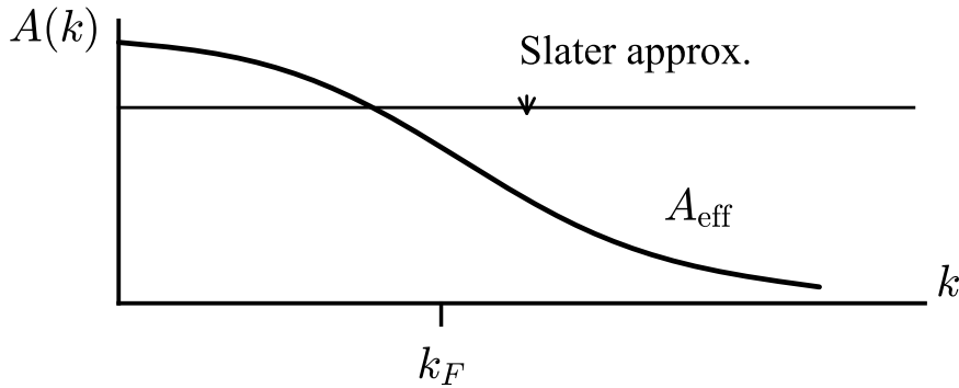
图 14 交换势 A(k) 与屏蔽后的 A_{\text{eff}} 随 k 的变化，水平线为 Slater 近似， k_F 处的奇性已被抹平（原书图注仅作“Figure 14”）
