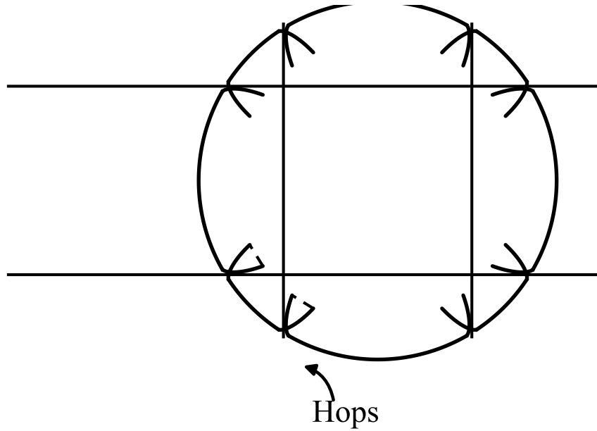
图 25 磁击穿示意：近自由电子的恒能轨道（圆）被区边界（直线网格）截断，电子绕轨道运行经过交点时跳跃（Hops）进入相邻轨道（原书图注仅作“Figure 25”）
