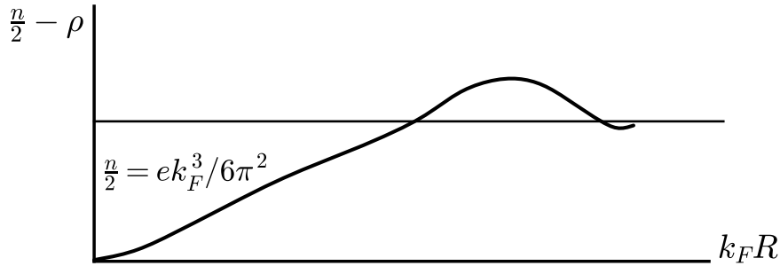
图 12 交换空穴：位于原点的电子周围自旋平行电子的总有效密度 n/2 - \rho 随 k_F R 的变化，水平线标记 n/2 = ek_F^3 / 6\pi^2 （原书图注仅作“Figure 12”）
