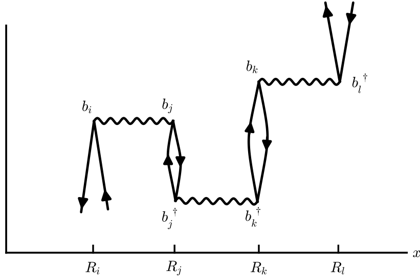
图 52 “反向图”示意：电子与空穴的径迹在 R_i 、 R_j 、 R_k 、 R_l 各处经波线相互作用，中间形成两个环状结构，各段标以 b_i 、 b_j 、 b_j^\dagger 、 b_k 、 b_k^\dagger 、 b_l^\dagger （原书图注仅作“Figure 52”）
