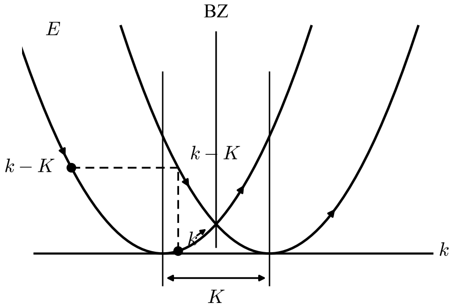
图 24 Zener 模型的 E - k 图：自由电子抛物线与其经倒格矢 K 平移的副本在区边界（竖直的 BZ 线）处交叉； k 与 k - K 两个加速态的轨迹（箭头）沿各自抛物线向上移动，底边双箭头标出间距 K （原书图注仅作“Figure 24”）
