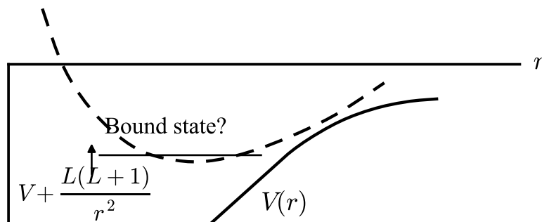
图 16 径向方程中势能项的草图：实线为 V(r) ，虚线为离心势 V + \frac{L(L+1)}{r^2} ，其谷底处标有“Bound state?”（束缚态？）（原书图注仅作“Figure 16”）
