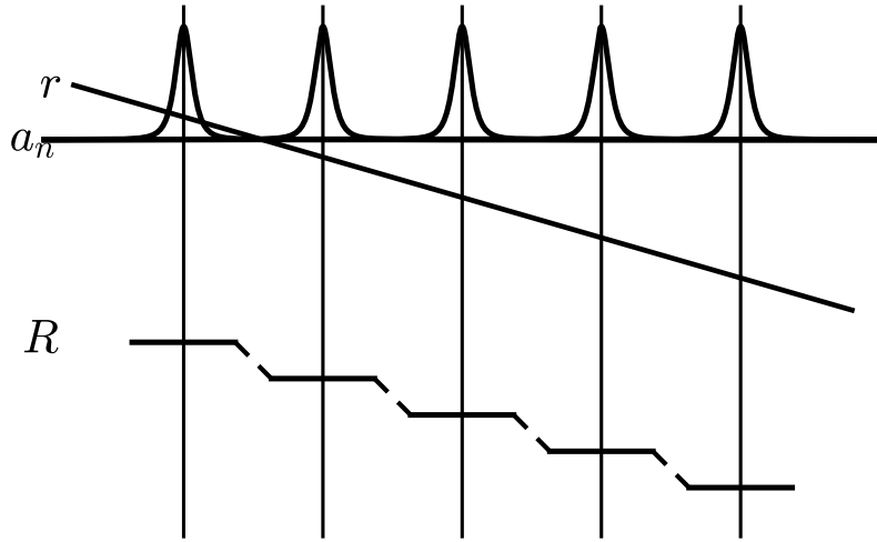
图 27 强局域情形下的线性势与阶梯势：自上而下依次为各格点上的 Wannier 函数 a_n （钟形峰）、线性势 r （斜直线）与阶梯下降的 R （平台之间以虚线相连），竖直线标记各格点位置（原书图注仅作“Figure 27”）
