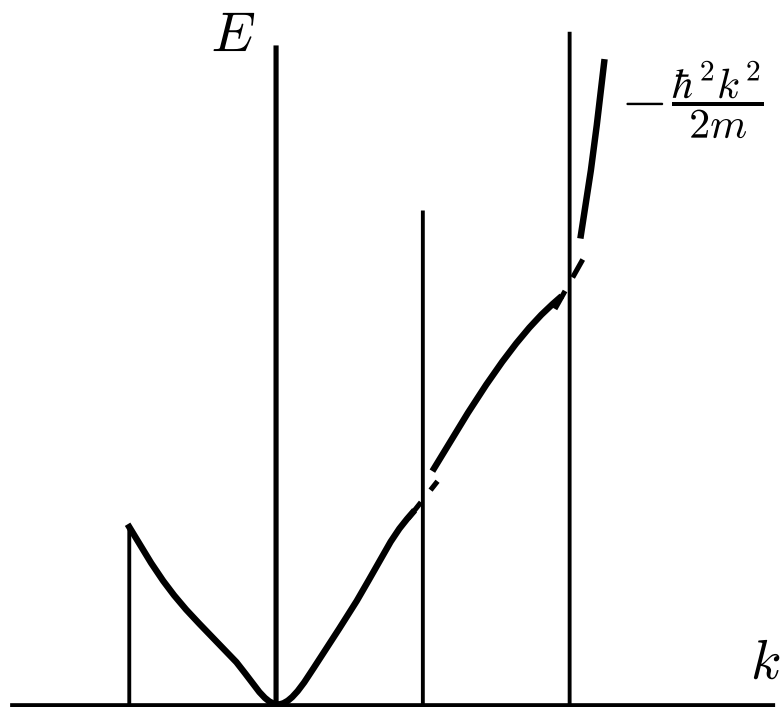
图 4 (原书图注仅 “ Figure 4 ” : E - k 曲线整体草图, 自由电子抛物线在各区边界处张开隙; 图中标注 -\hbar^2 k^2/2m )
