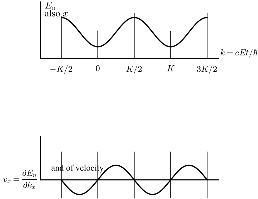
图 19 E_n (亦即位置 x ) 随 k = eEt/\hbar 的周期性变化 (横轴标出 -K/2 、 0 、 K/2 、 K 、 3K/2 )，以及速度 v_x = \partial E_n / \partial k_x 随时间的对应周期性变化 (原书图注仅作“Figure 19”)
