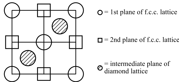
图 6 金刚石格子。○ = f.c.c. 格子的第一平面；□ = f.c.c. 格子的第二平面；斜纹圆 = 金刚石格子的中间平面
