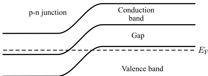
图 21 p-n 结的能带图：导带（Conduction band）、禁带（Gap）与价带（Valence band）在结区弯曲衔接，虚线为费米面 E_F （原书图注仅作“Figure 21”）
