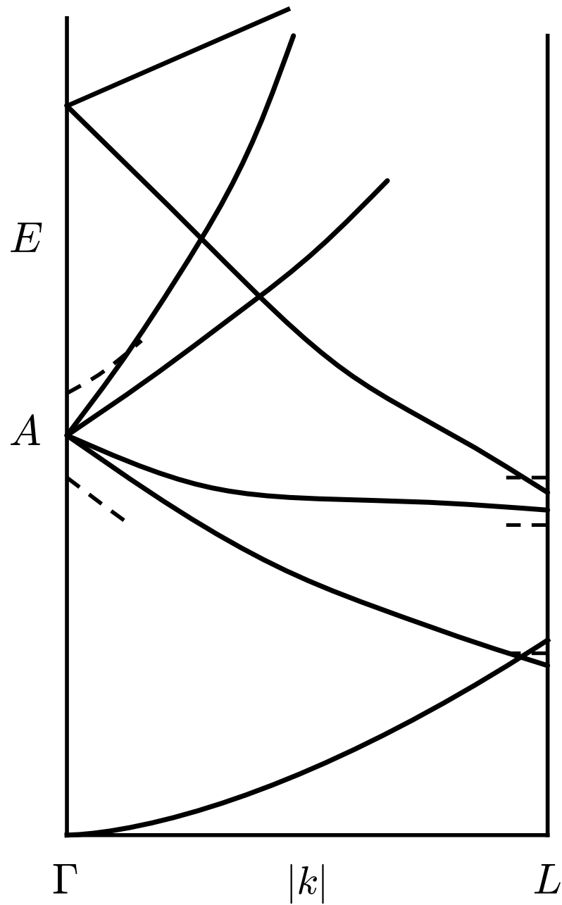
图 5 f.c.c. 空间格子沿从原点到区边界六边形面的直线（即 k = (x, x, x) 方向）的能量对 k 曲线（自由电子抛物面折回简约区后的结果）
