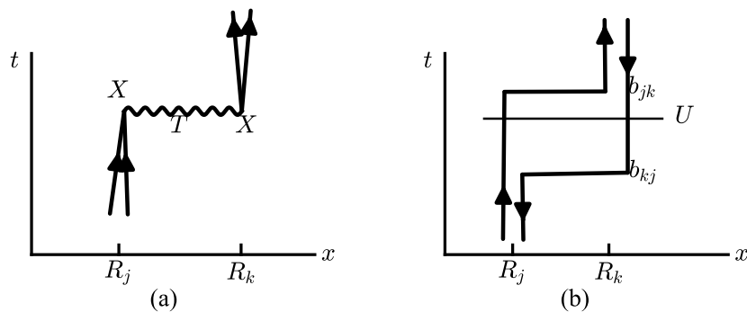
图 49 t - x 图两种情形：(a) 电子与空穴的径迹在 R_j 与 R_k 处各标一次 “X”，其间由标 “T” 的波线相连，两端各有向上的箭头；(b) 虚跳图：标 b_{jk} 与 b_{kj} 的竖直跳变跨过标 U 的水平线 (原书图注仅作 “Figure 49”)
