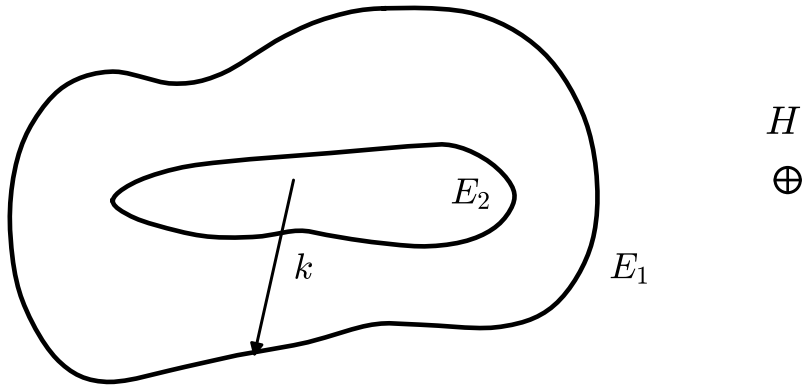
图 22 磁场中的恒能面与轨道: 两条闭合恒能线 E_1 与 E_2 , \mathbf{k} 沿等能线绕行 (箭头), \mathbf{H} 垂直于纸面 (图中以 \oplus 标出) (原书图注仅作“Figure 22”)
