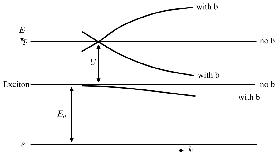
图 46 能级示意：p 能级与激子（Exciton）能级各给出 no b（不计 b ，水平直线）与 with b（计入 b ，曲线）两种情形； U 标出 p 组态与激子组态之间的能量间隔， E_0 为自 s 能级到激子能级的间距，左侧箭头 E 指示能量向下减小，横轴为 k （原书图注仅作“Figure 46”）
