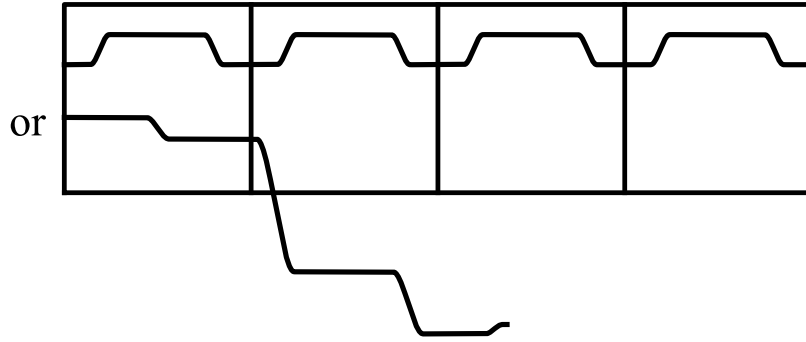
图 23 开放轨道示意：扩展区图式中的恒能线，“or”连出两种情形——或者在每个区内闭合，或者穿越一个又一个区边界延伸出去（原书图注仅作“Figure 23”）
