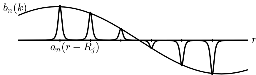
图 26 紧束缚 Bloch 波函数实部示意：缓变的 b_n(k) 乘以各格点上的 Wannier 函数 a_n(r - R_j) （钟形峰），过零后峰反号；横轴为 r （原书图注仅作“Figure 26”）
