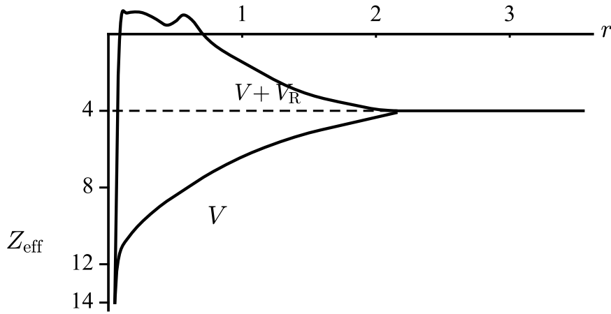
图 15 Si 中势的抵消: V 与 V + V_R 的有效电荷 Z_{\text{eff}} 随 r 的变化 (纵轴刻度自上而下为 4、8、12、14), V 在芯区内深达 14, V + V_R 很快趋于虚线所示的约 4 的浅势; 横轴 r 标 1、2、3 (原书图注仅作 “Figure 15”)
